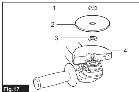
Fig.17 ► 1. Contre-écrou 2. Meule tronçonneuse abrasive / meule diamant 3. Flasque intérieur 4. Protecteur de meule pour meule tronçonneuse abrasive / meule diamant
